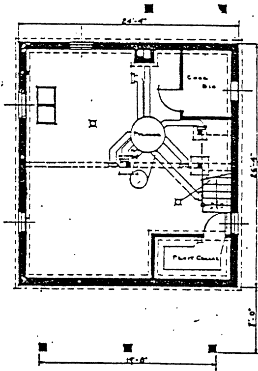
BASEMENT-PLAN.
