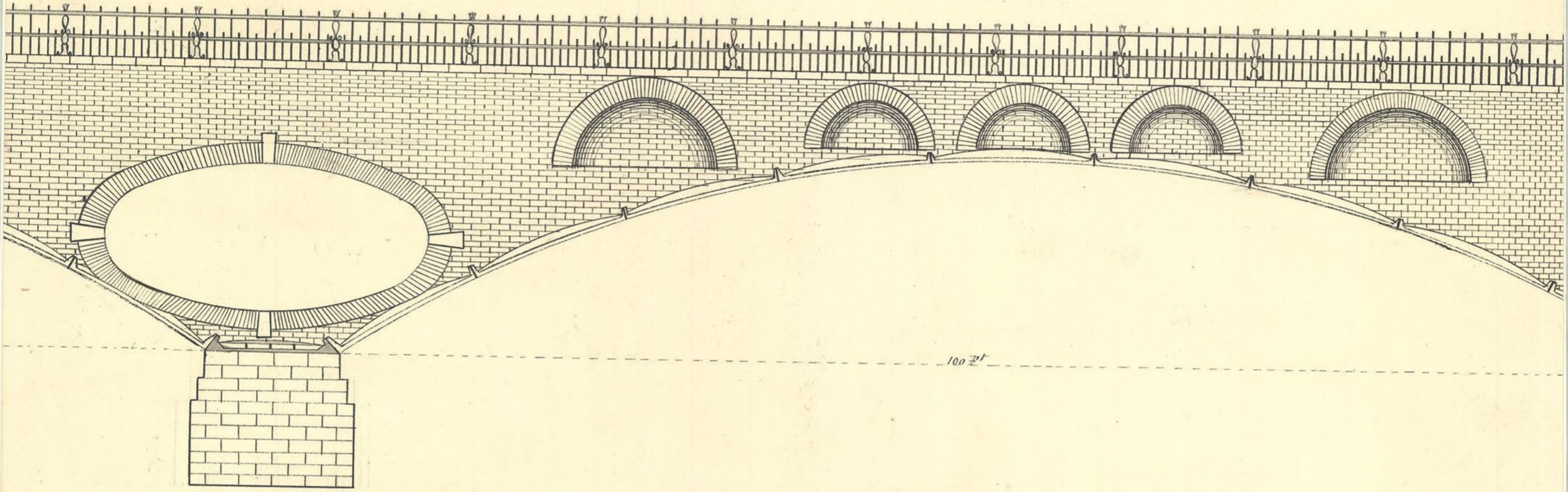
Elevation
